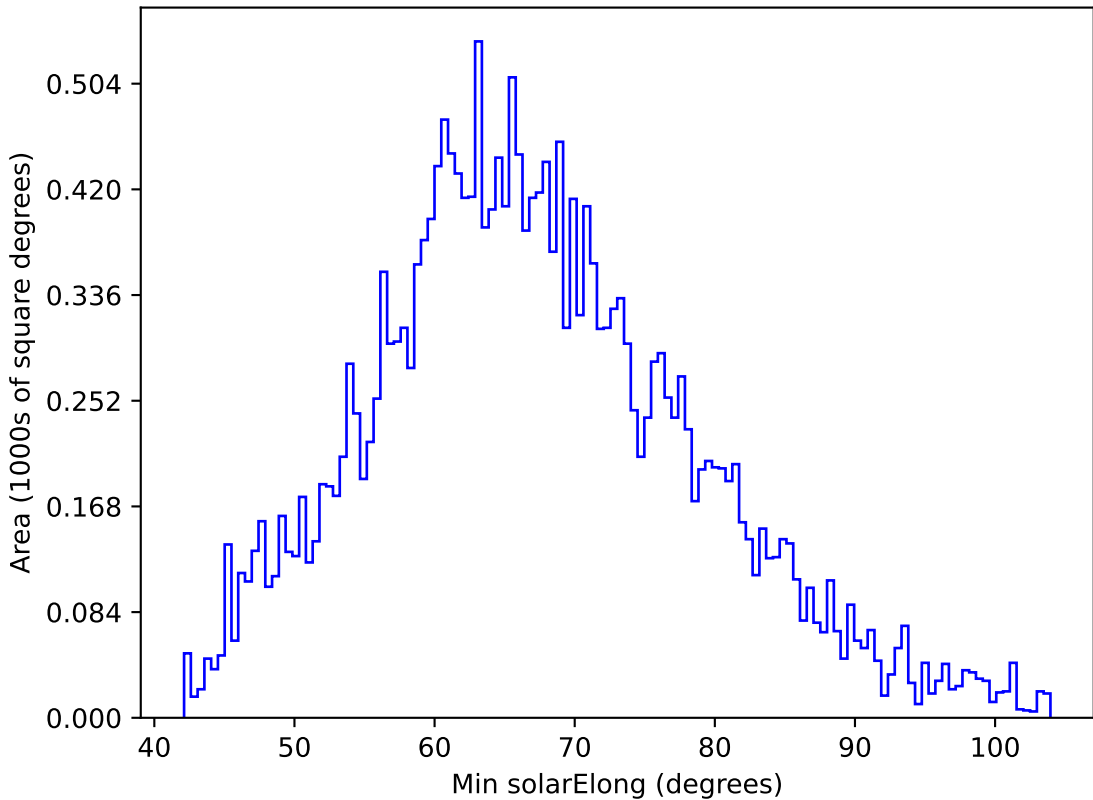
ddf_acor_sf20_lsf0_lsr0_v3.4_10yrs All sky y band: Min solarElong
