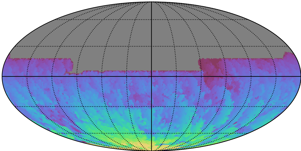
ddf_acor_sf20_lsf0_lsr0_v3.4_10yrs All sky y band: Max HA
