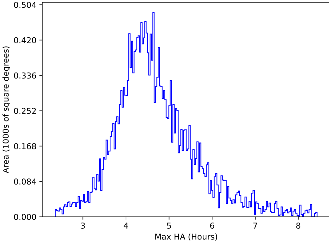
ddf_acor_sf20_lsf0_lsr0_v3.4_10yrs All sky y band: Max HA
