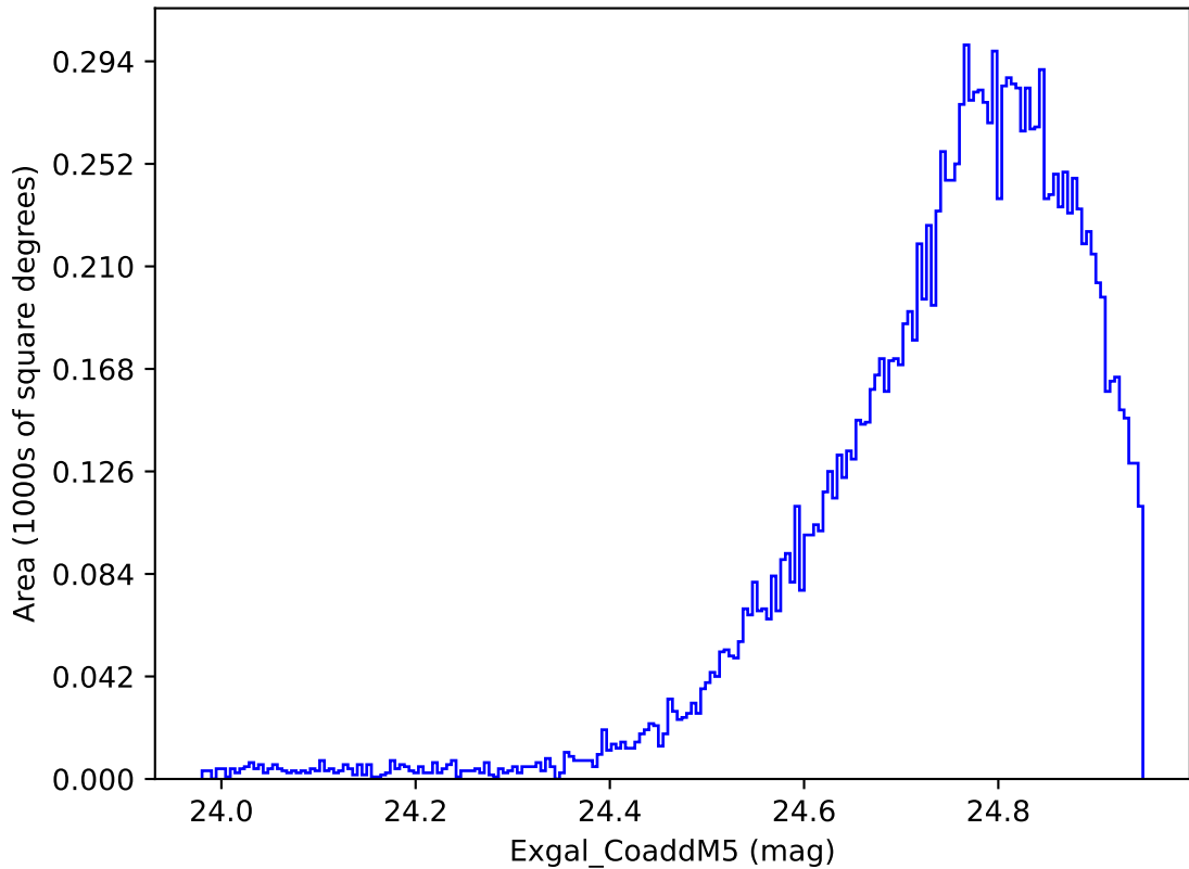
ddf_acor_sf20_lsf0_lsr0_v3.4_10yrs WFD y band: Exgal_CoaddM5
