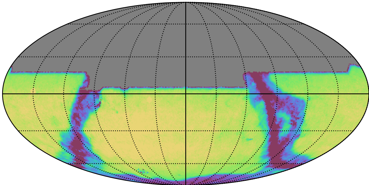
ddf_acor_sf20_lsf0_lsr0_v3.4_10yrs All sky y band: Exgal_CoaddM5
