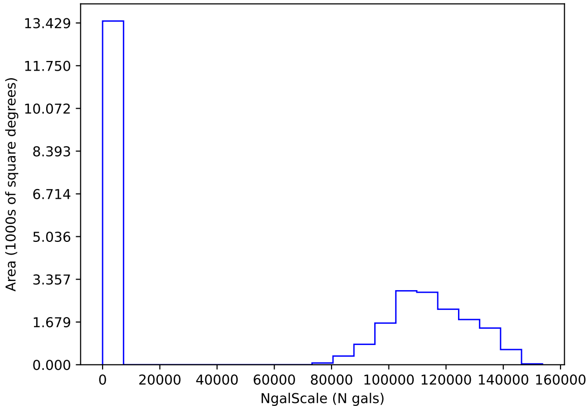
ddf_acor_sf15_lsf40_lsr50_v3.4_10yrs i: NgalScale
