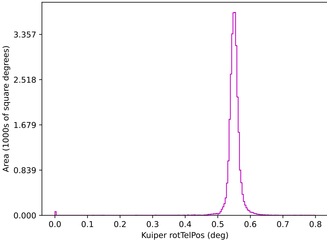
ddf_acor_sf15_lsf40_lsr50_v3.4_10yrs z: Kuiper rotTelPos
