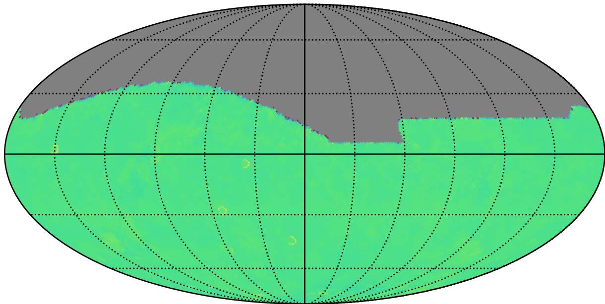
ddf_acor_sf15_lsf40_lsr50_v3.4_10yrs i: Kuiper rotTelPos
