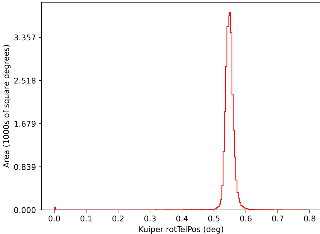
ddf_acor_sf15_lsf40_lsr50_v3.4_10yrs i: Kuiper rotTelPos
