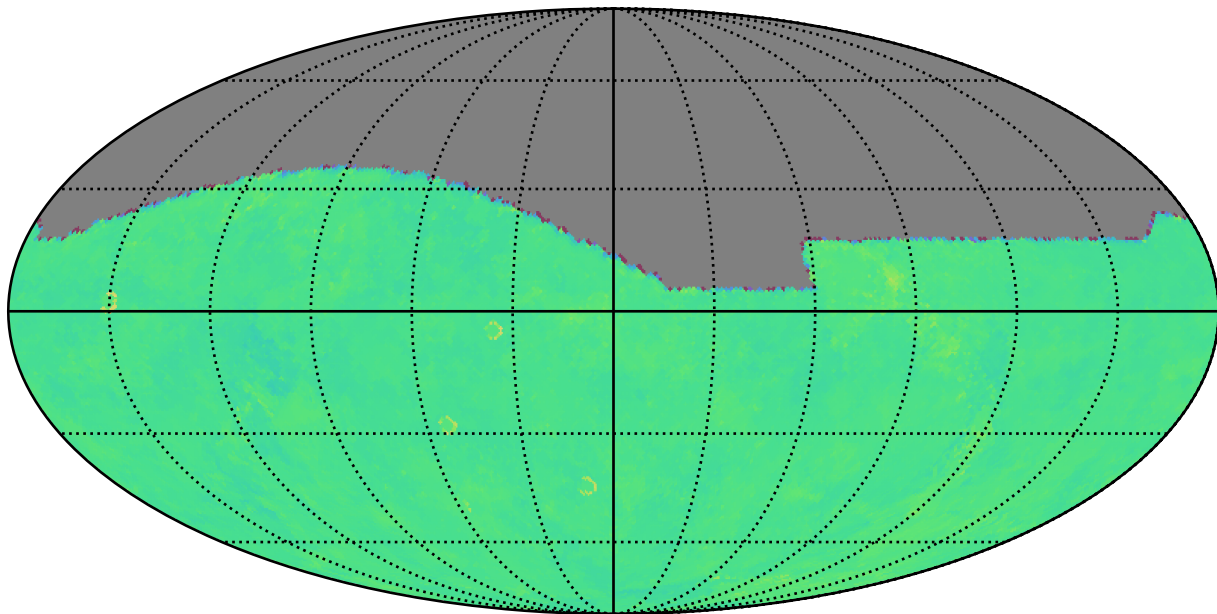
ddf_acor_sf15_lsf40_lsr50_v3.4_10yrs g: Kuiper rotTelPos
