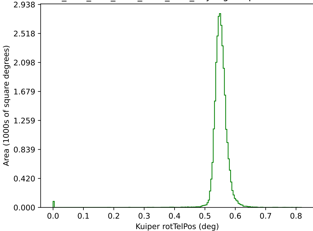
ddf_acor_sf15_ls40_lsr50_v3.4_10yrs g: Kuiper rotTelPos
