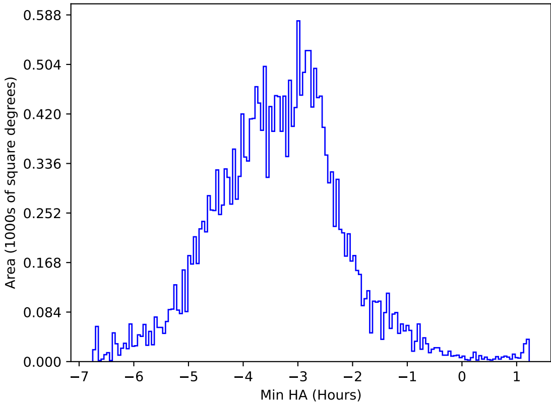
ddf_acor_sf15_ls40_lsr50_v3.4_10yrs All sky y band: Min HA
