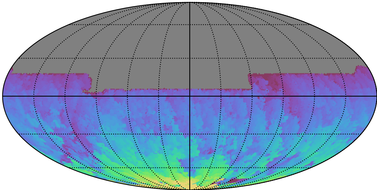
ddf_acor_sf15_lsf40_lsr50_v3.4_10yrs All sky y band: Max HA
