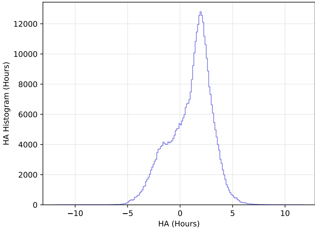
ddf_acor_sf15_lsf40_lsr50_v3.4_10yrs All sky y band: HA Histogram
