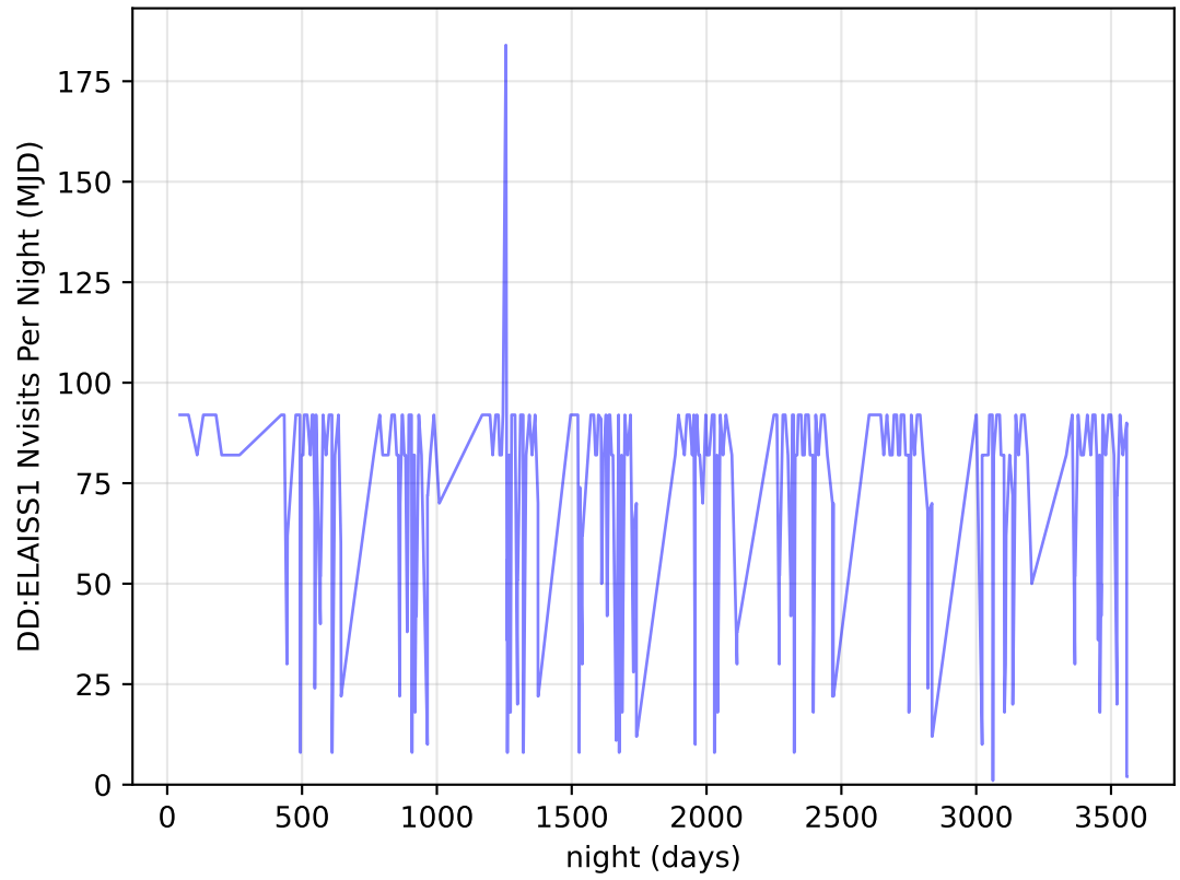
ddf_acor_sf15_lsf40_lsr50_v3.4_10yrs all bands: DD:ELAISS1 Nvisits Per Night
