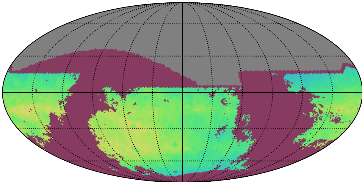
ddf_acor_sf15_lsf40_lsr20_v3.4_10yrs i: NgalScale
