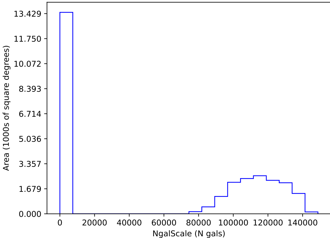
ddf_acor_sf15_lsf40_lsr20_v3.4_10yrs i: NgalScale
