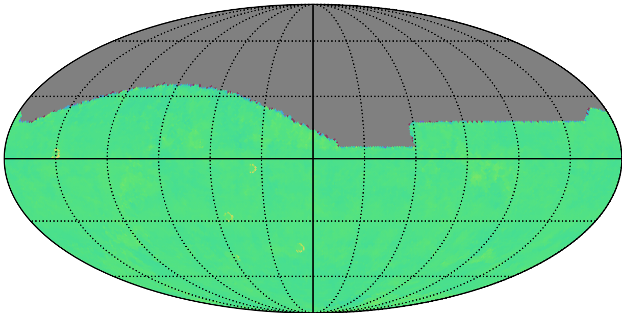
ddf_acor_sf15_lsf40_lsr20_v3.4_10yrs i: Kuiper rotTelPos
