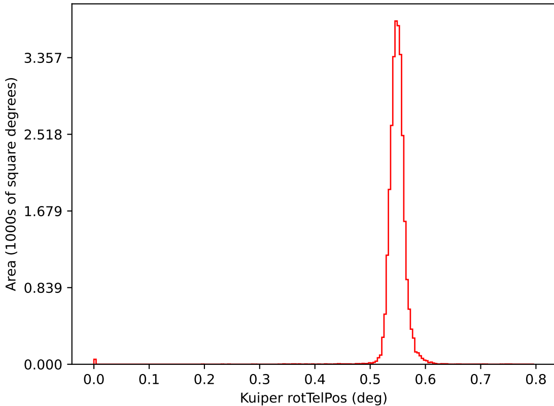
ddf_acor_sf15_lsf40_lsr20_v3.4_10yrs i: Kuiper rotTelPos
