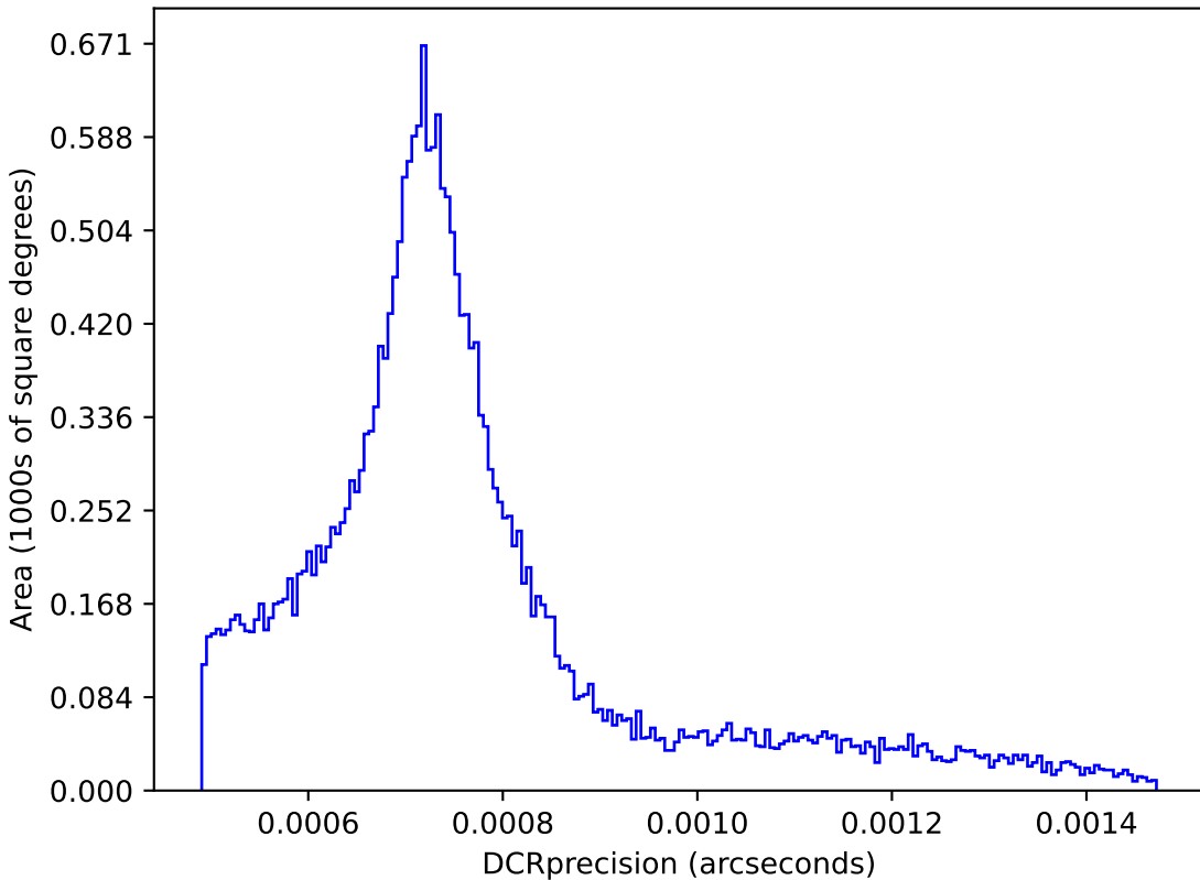
ddf_acor_sf15_lsf40_lsr20_v3.4_10yrs : DCRprecision
