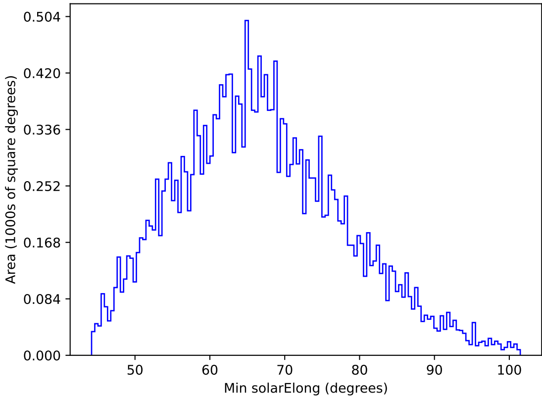
ddf_acor_sf15_lsf40_lsr20_v3.4_10yrs All sky y band: Min solarElong
