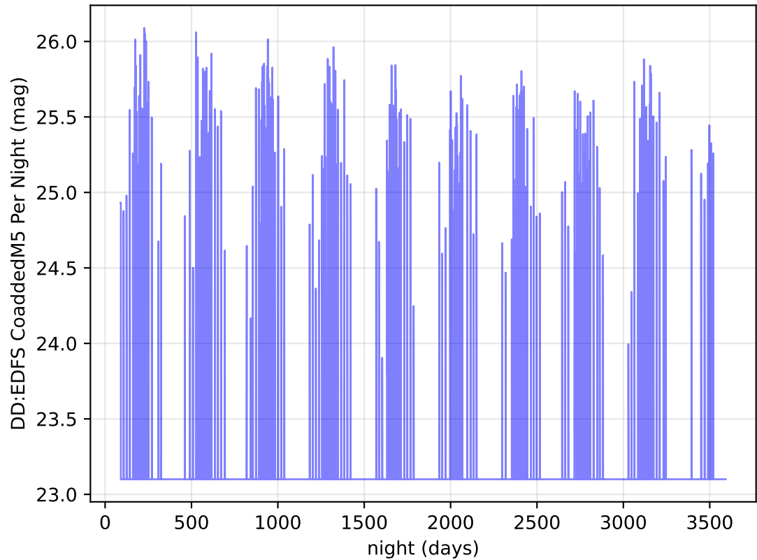
ddf_acor_sf15_Isf40_Isr20_v3.4_10yrs i band: DD:EDFS CoaddedM5 Per Night
