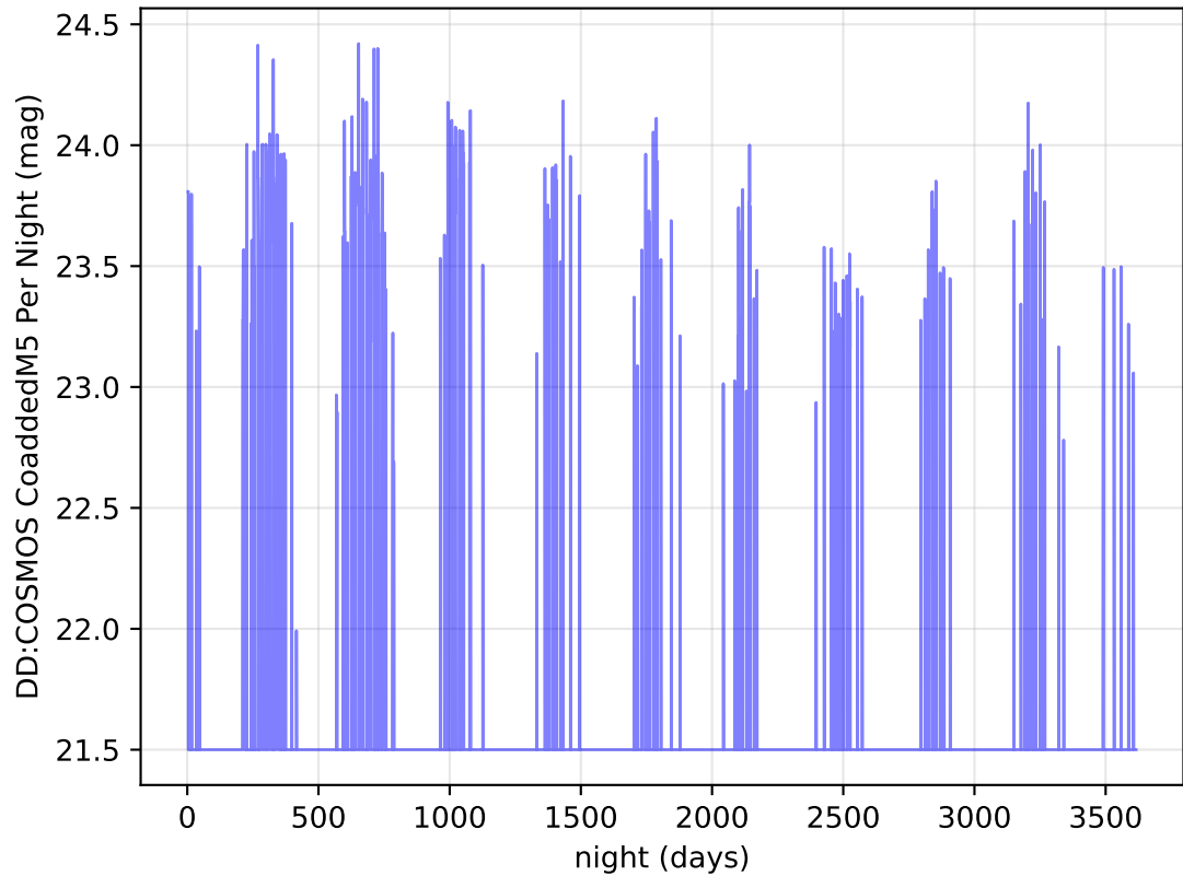
ddf_acor_sf15_lsf40_lsr20_v3.4_10yrs y band: DD:COSMOS CoaddedM5 Per Night
