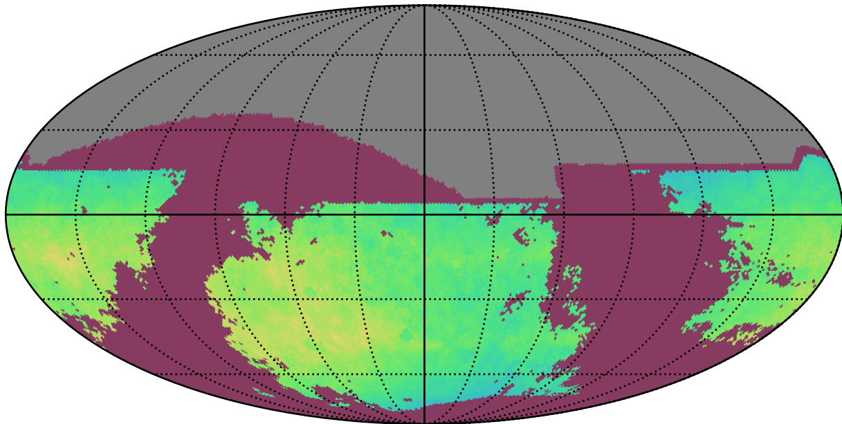
ddf_acor_sf15_lsf40_lsr10_v3.4_10yrs i: NgalScale
