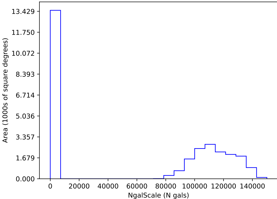
ddf_acor_sf15_lsf40_lsr10_v3.4_10yrs i: NgalScale
