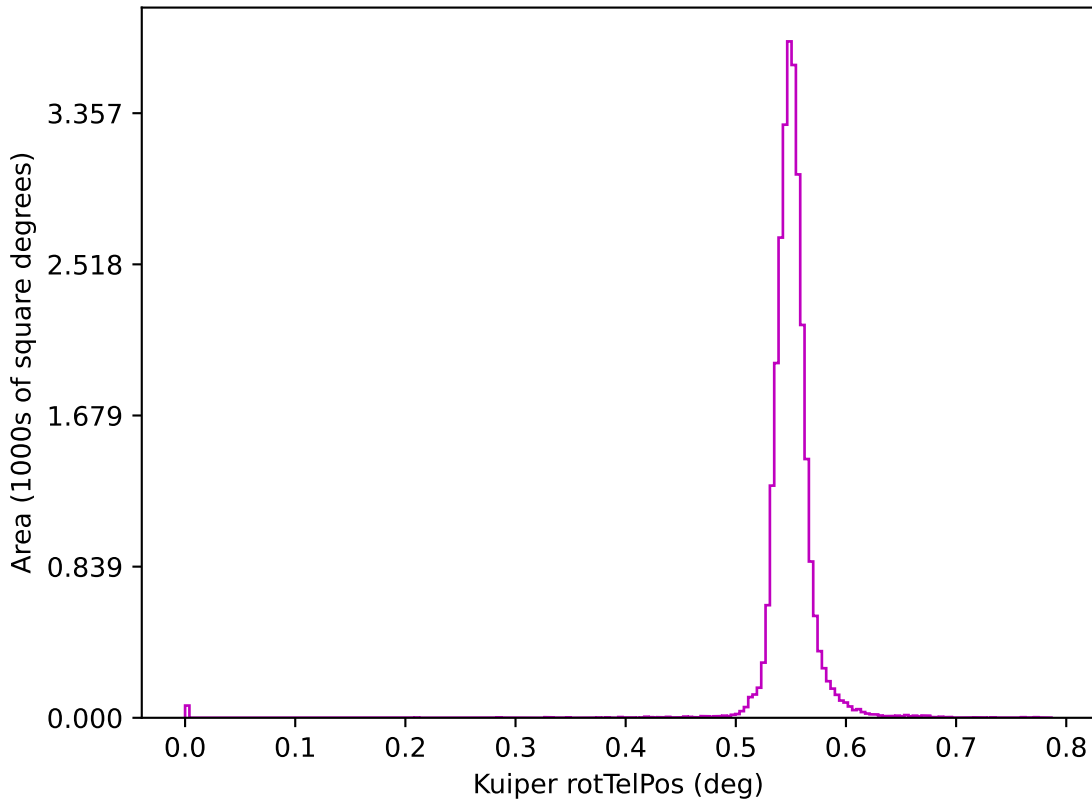
ddf_acor_sf15_lsf40_lsr10_v3.4_10yrs z: Kuiper rotTelPos
