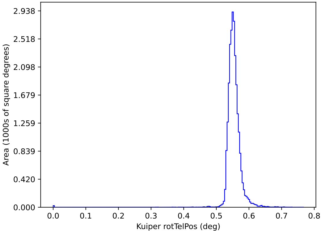
ddf_acor_sf15_lsf40_lsr10_v3.4_10yrs y: Kuiper rotTelPos
