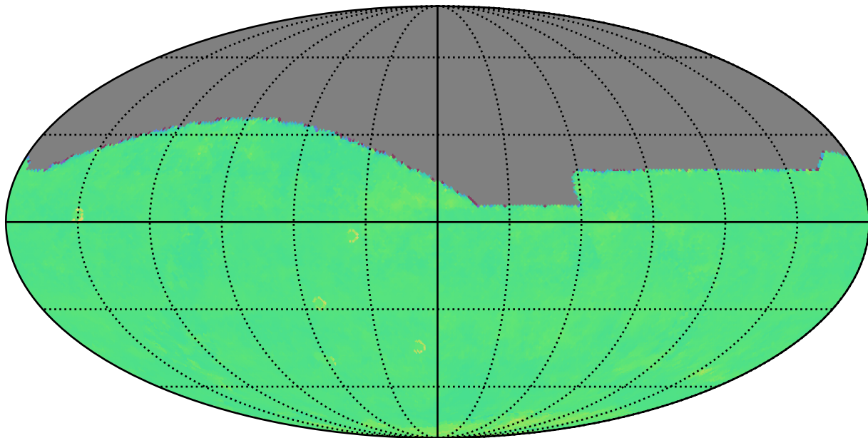
ddf_acor_sf15_lsf40_lsr10_v3.4_10yrs r: Kuiper rotTelPos
