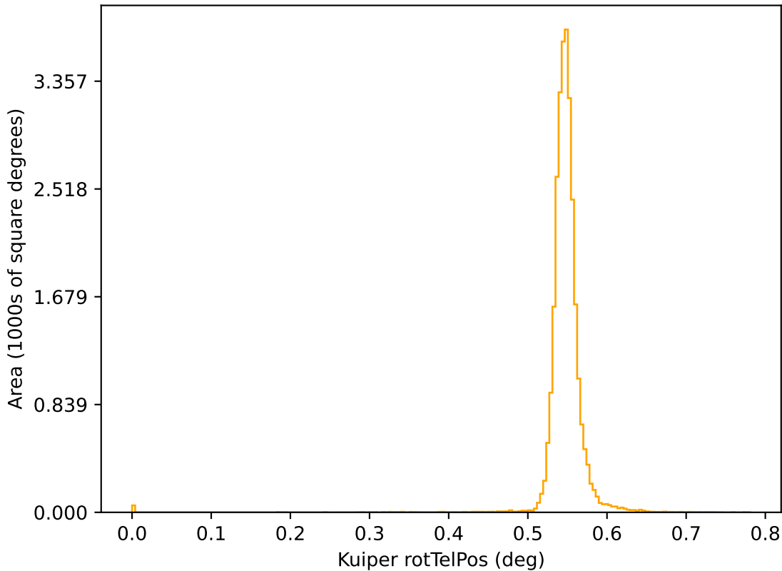
ddf_acor_sf15_lsf40_lsr10_v3.4_10yrs r: Kuiper rotTelPos
