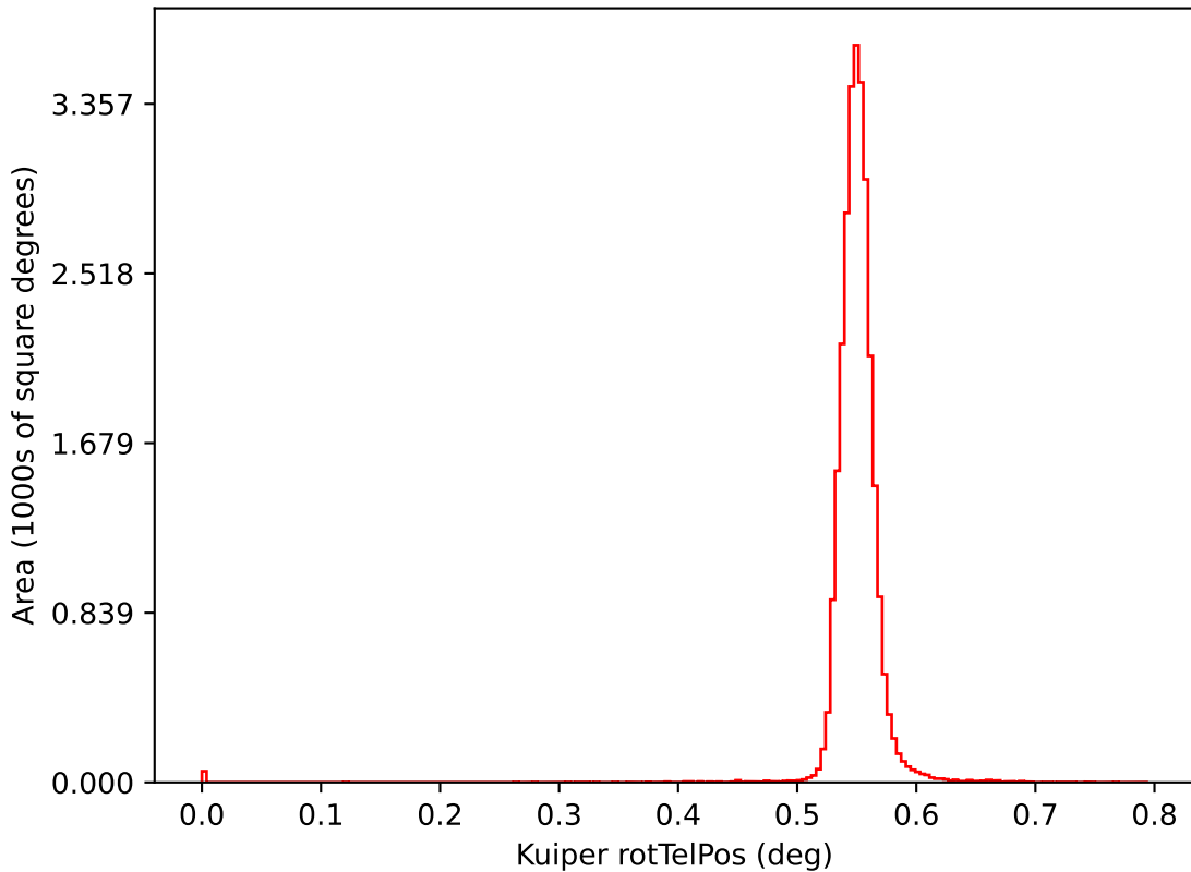
ddf_acor_sf15_lsf40_lsr10_v3.4_10yrs i: Kuiper rotTelPos
