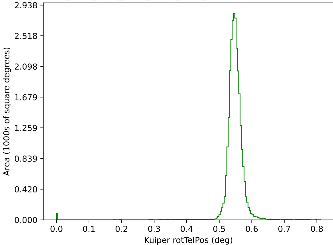
ddf_acor_sf15_ls40_lsr10_v3.4_10yrs g: Kuiper rotTelPos
