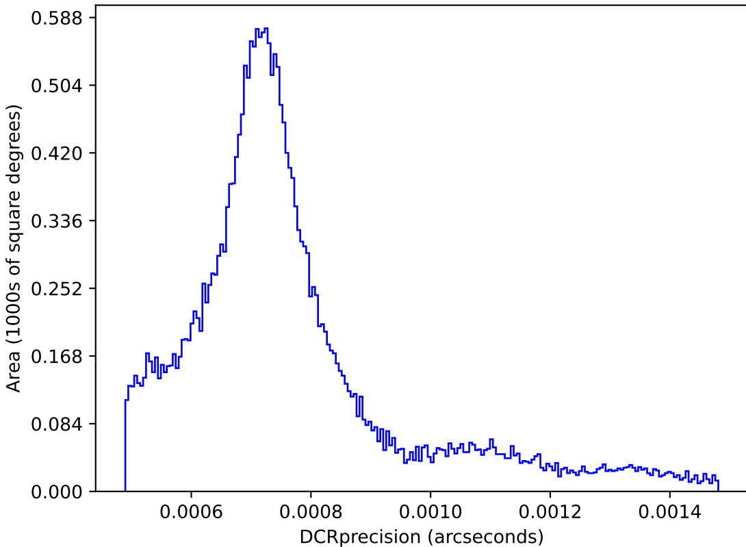
ddf_acor_sf15_lsf40_lsr10_v3.4_10yrs : DCRprecision
