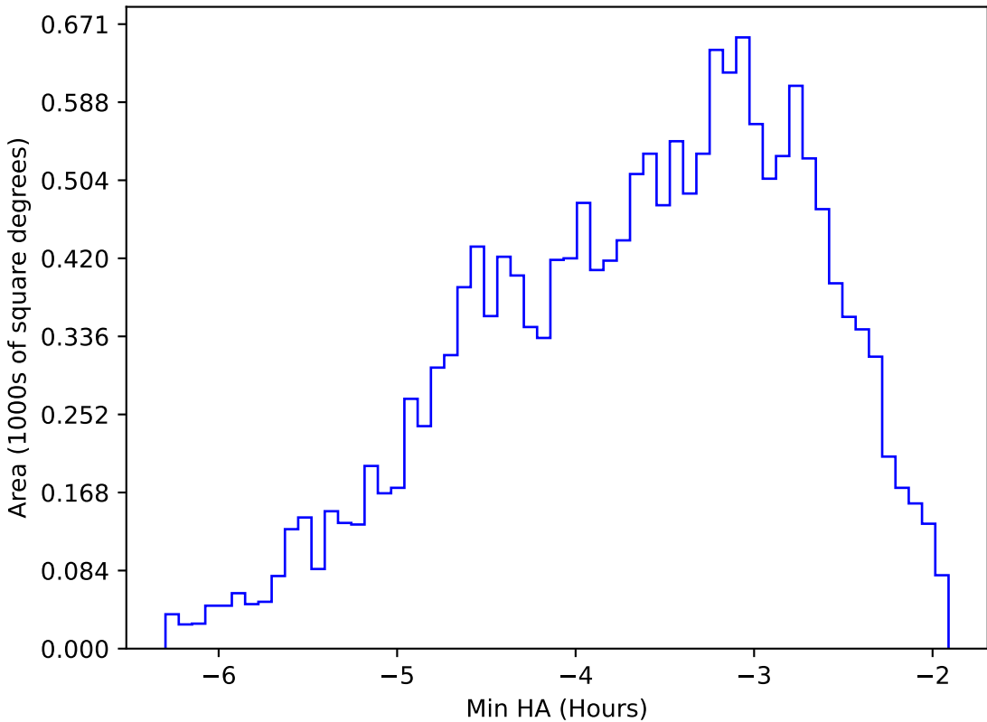
ddf_acor_sf15_lsf40_lsr10_v3.4_10yrs WFD y band: Min HA
