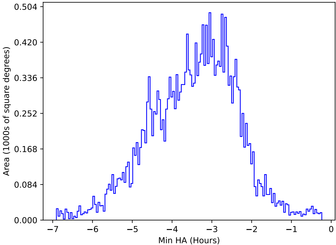
ddf_acor_sf15_lsf40_lsr10_v3.4_10yrs All sky y band: Min HA
