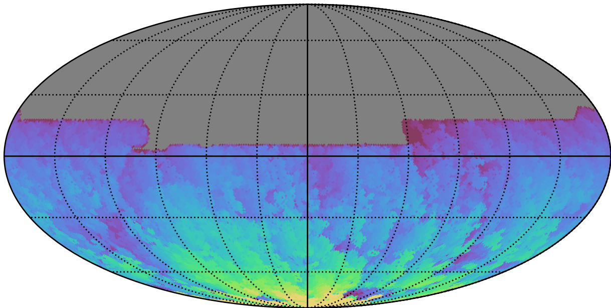
ddf_acor_sf15_lsf40_lsr10_v3.4_10yrs All sky y band: Max HA
