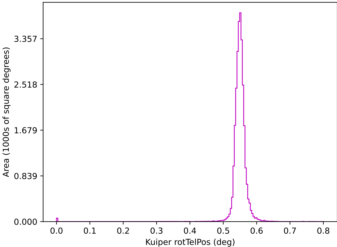
ddf_acor_sf15_lsf30_lsr50_v3.4_10yrs z: Kuiper rotTelPos
