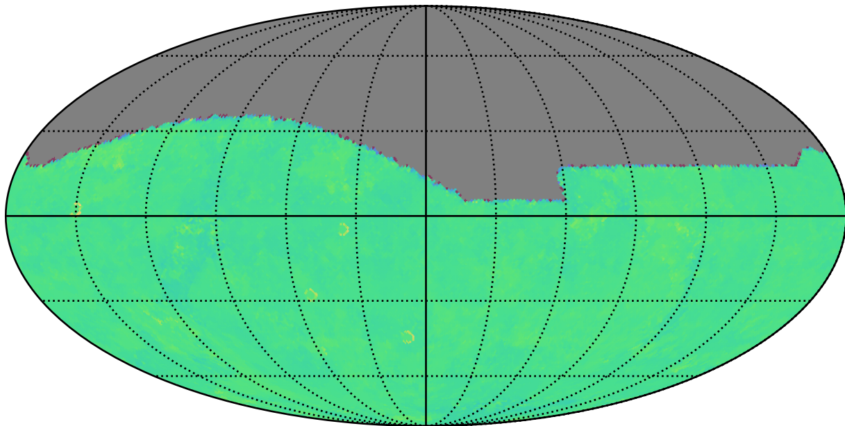
ddf_acor_sf15_lsf30_lsr50_v3.4_10yrs g: Kuiper rotTelPos
