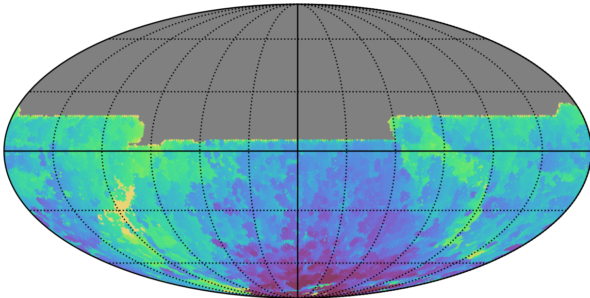
ddf_acor_sf15_lsf30_lsr50_v3.4_10yrs All sky y band: Min HA
