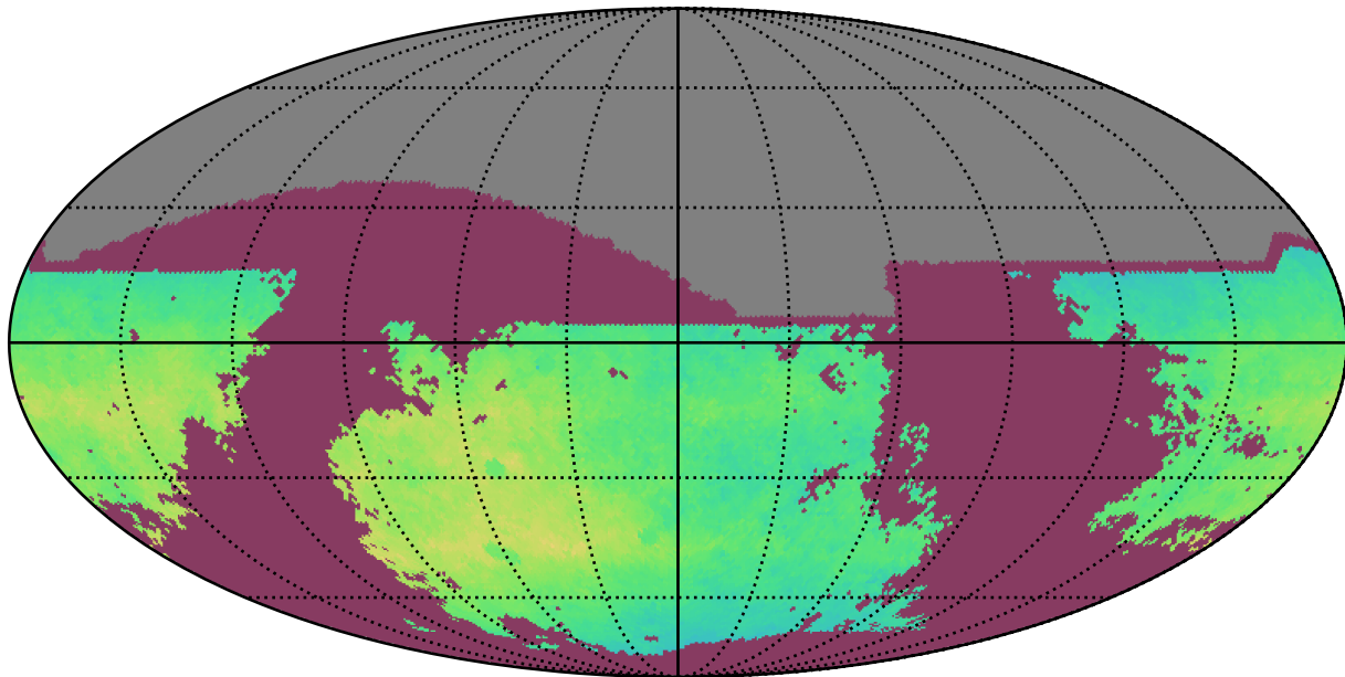
ddf_acor_sf15_lsf30_lsr20_v3.4_10yrs i: NgalScale
