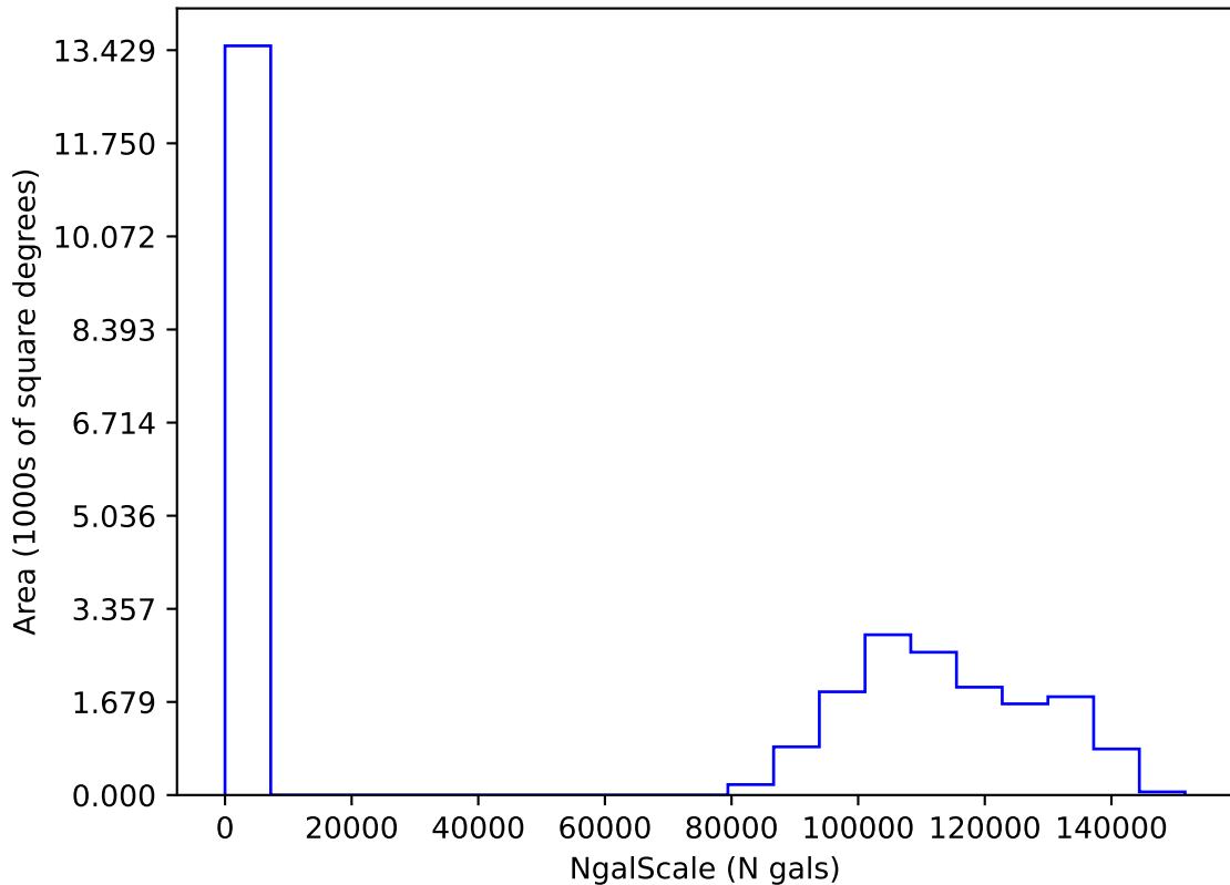
ddf_acor_sf15_lsf30_lsr20_v3.4_10yrs i: NgalScale
