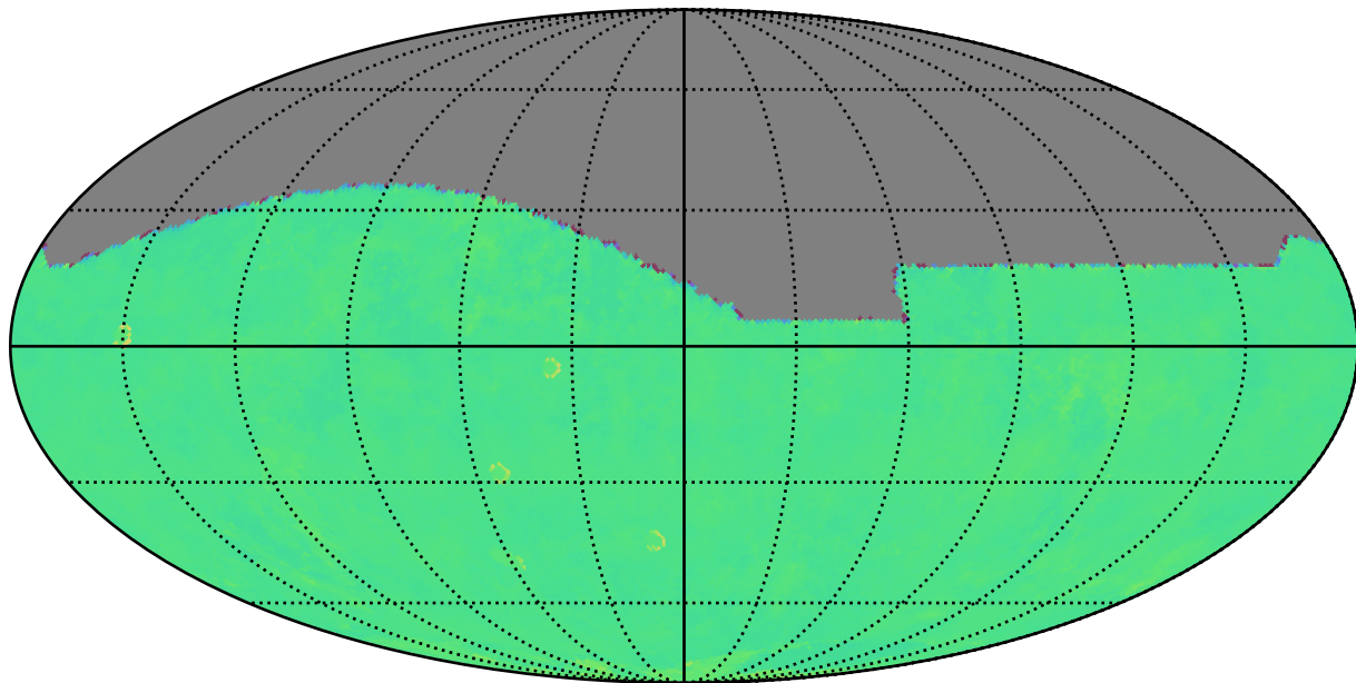
ddf_acor_sf15_lsf30_lsr20_v3.4_10yrs i: Kuiper rotTelPos
