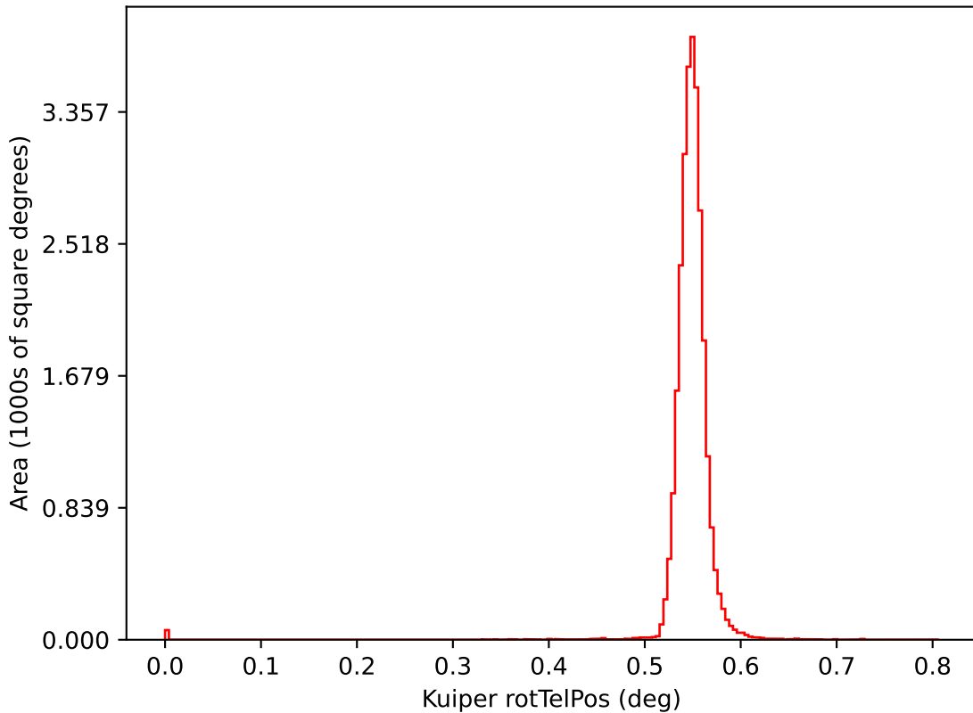
ddf_acor_sf15_lsf30_lsr20_v3.4_10yrs i: Kuiper rotTelPos
