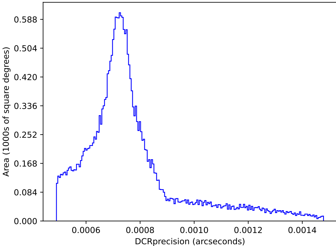
ddf_acor_sf15_lsf30_lsr20_v3.4_10yrs : DCRprecision
