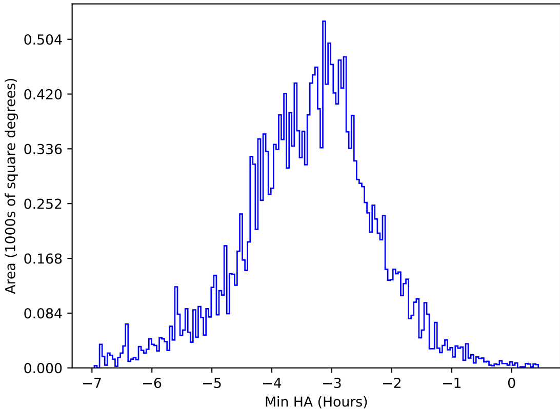
ddf_acor_sf15_lsf30_lsr20_v3.4_10yrs All sky y band: Min HA
