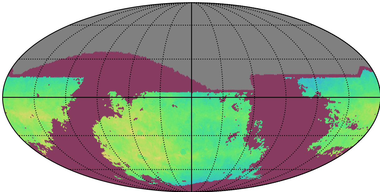
ddf_acor_sf15_lsf30_lsr10_v3.4_10yrs i: NgalScale
