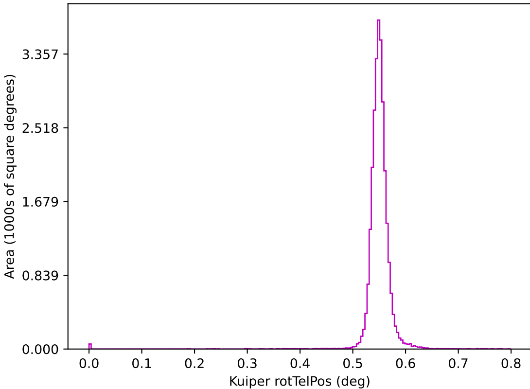
ddf_acor_sf15_lsf30_lsr10_v3.4_10yrs z: Kuiper rotTelPos
