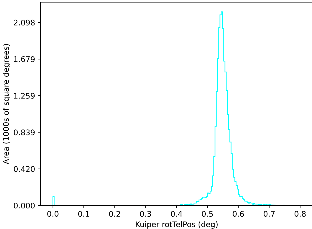
ddf_acor_sf15_ls30_lsr10_v3.4_10yrs u: Kuiper rotTelPos
