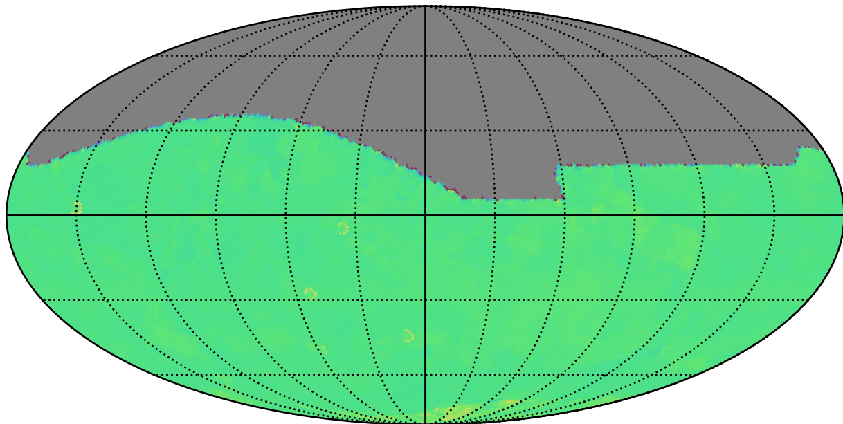
ddf_acor_sf15_lsf30_lsr10_v3.4_10yrs r: Kuiper rotTelPos
