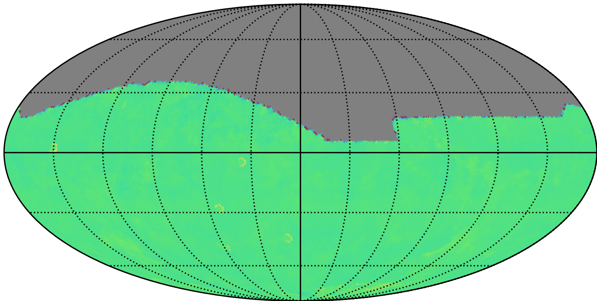
ddf_acor_sf15_lsf30_lsr10_v3.4_10yrs i: Kuiper rotTelPos
