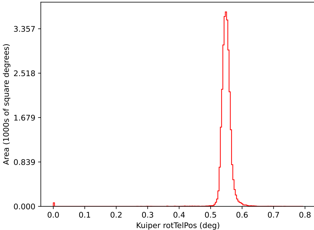
ddf_acor_sf15_lsf30_lsr10_v3.4_10yrs i: Kuiper rotTelPos
